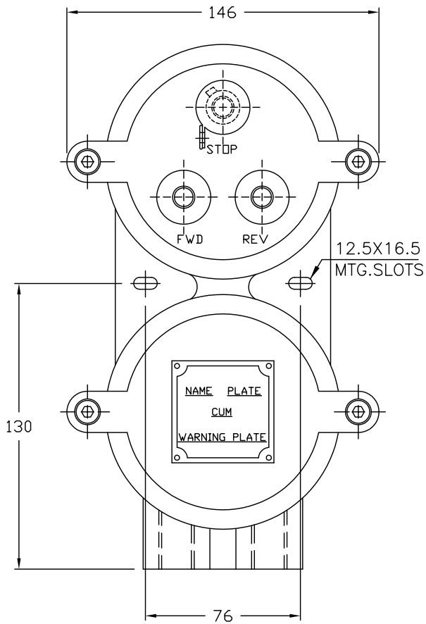
ELEVATION
